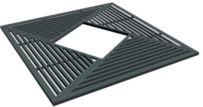
Uno TS-01 • length - 1800 mm • width - 1800 mm • height - 50 mm • hole - 700×700 mm
