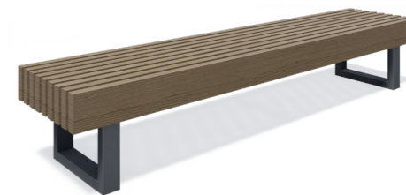
Colt BN-03 • length - 2500 mm • width - 520 mm • height - 440 mm
